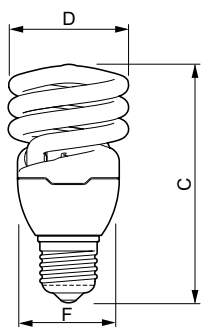
TORNADO 20W CDL E27 220-240V 50/60Hz
