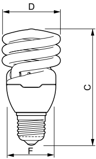
TORNADO 20W CDL E27 110-127V 50/60Hz
