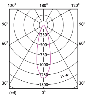
LEDspots PL 4,9W PAR20 E27 827 25D
