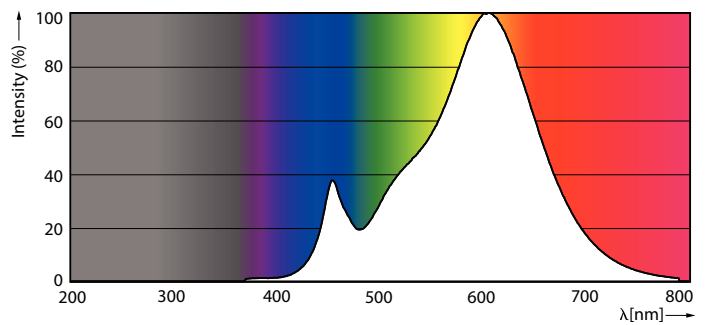
LEDspots K 50W PAR16 GU10 827 36D-POC
