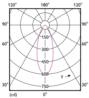
LEDspots K 50W PAR16 GU10 827 36D-LDD
