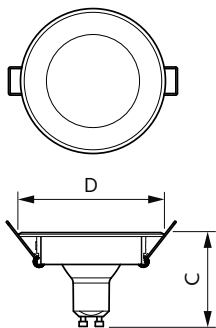
LEDspot50W GU10Kit_R 827 100-240V 36D
