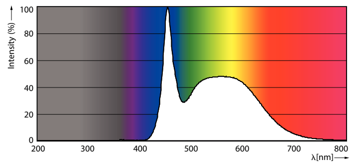
LEDbulb E27 A25
