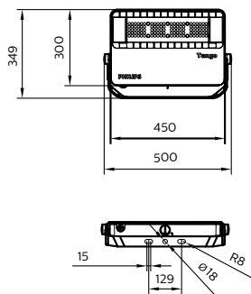
BVP38x Tango G3
