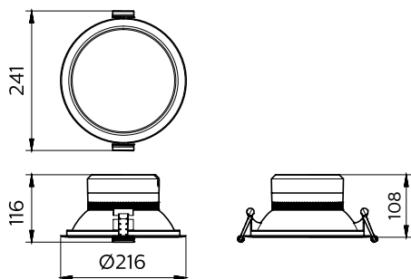
DN392B LED16/830 PSU D200 ALU GM
