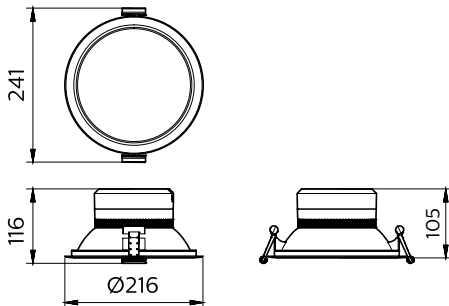
DN392B LED16/840 PSU D200 WH GM
